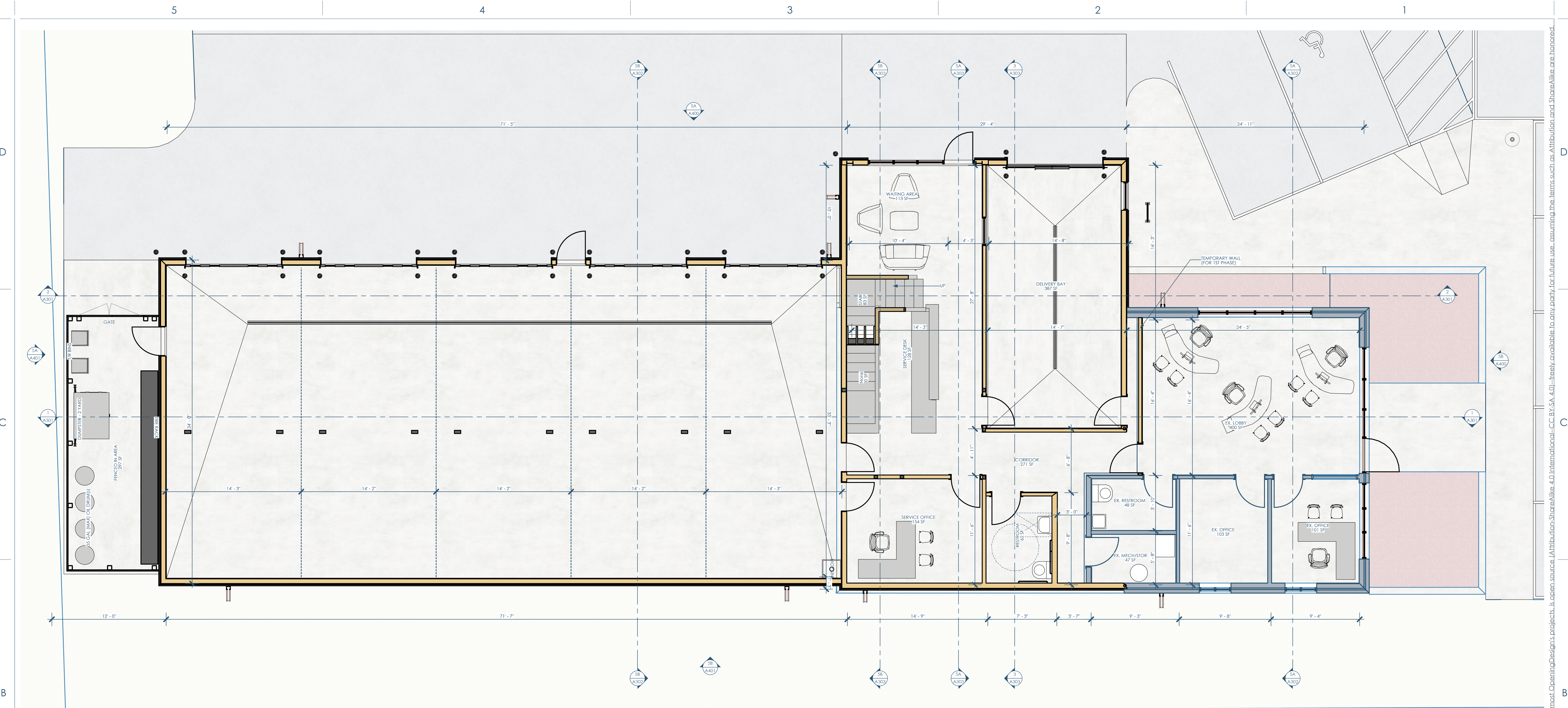
5B/A101_1 FOO PLAN 1/4"=1'-0"
